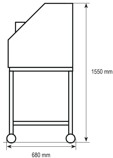
VUE LATÉRALE | SIDE VIEW | ZIJEAANZICHT
